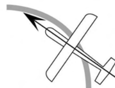
Nez pointant vers l'intérieur : Enlevez de la direction et/ou du différentiel d'aileron
